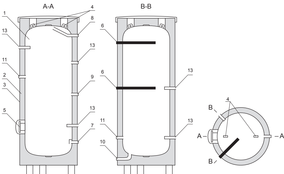
Rys. 1 Budowa zasobnika 750 l.
