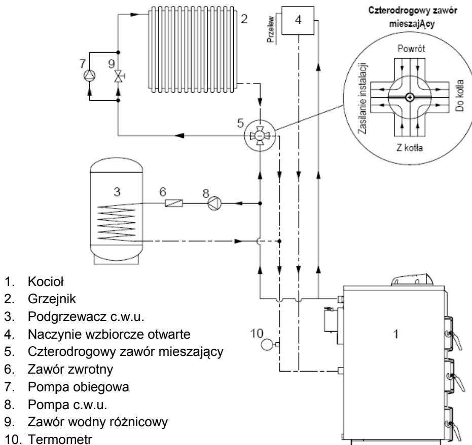
Rys.7. Przykładowy schemat podłączenia kotła do systemu grzewczego c.o. i c.w.u. z wykorzystaniem czterodrogowego zaworu mieszającego.
