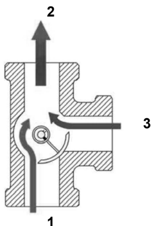
Rys. 6. Trójdrożny zawór mieszający
