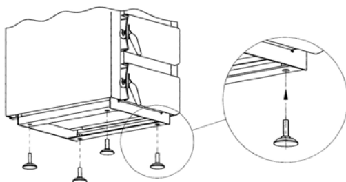
Rys.4 Poziomowanie kotła
