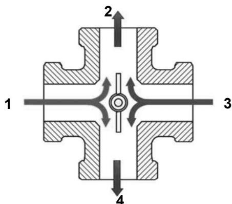
Rys.5. Czterodrożny zawór mieszający
