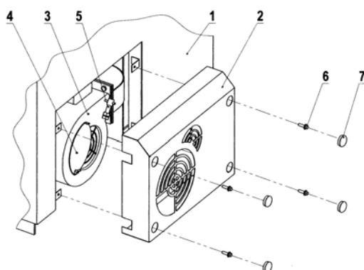
Rys.3 Wentylator nadmuchowy 1 – obudowa kotła 2 – osłona wentylatora 3 – wentylator nadmuchowy 4 – przysłona
