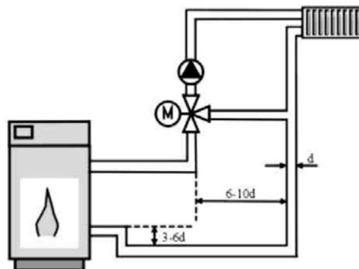
Przykład montażu zaworu mieszającego
