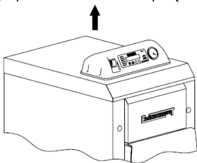
Rys. 9 Demontaż pokrywy obudowy kotła i przewodu termomanometru.
